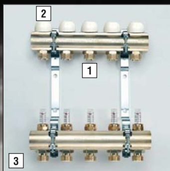
Art. TM 3856 rozdělovač pro podlahové vytápění - přívod G1" - připojení okruhů G3/4"x18 EUROCONUS - provedení 3856 verze s průtokoměry
