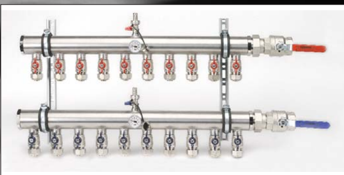
Art. TM 3920 plně osazený průmyslový nerezový rozdělovač pro podlahové vytápění - přívod G 2" - připojení okruhů G 1"
